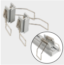
2 staffe di montaggio per incasso su cartongesso
