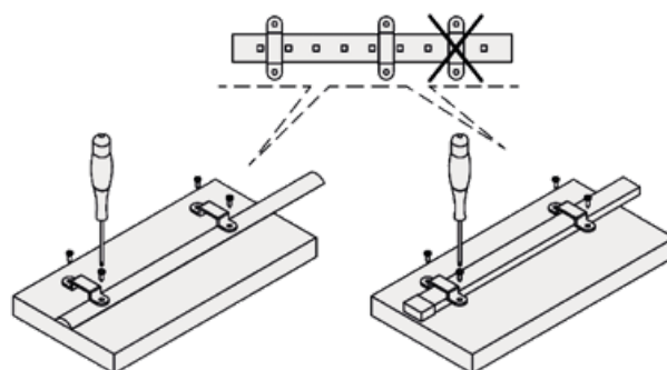
Installazione con biadesivo e clip
